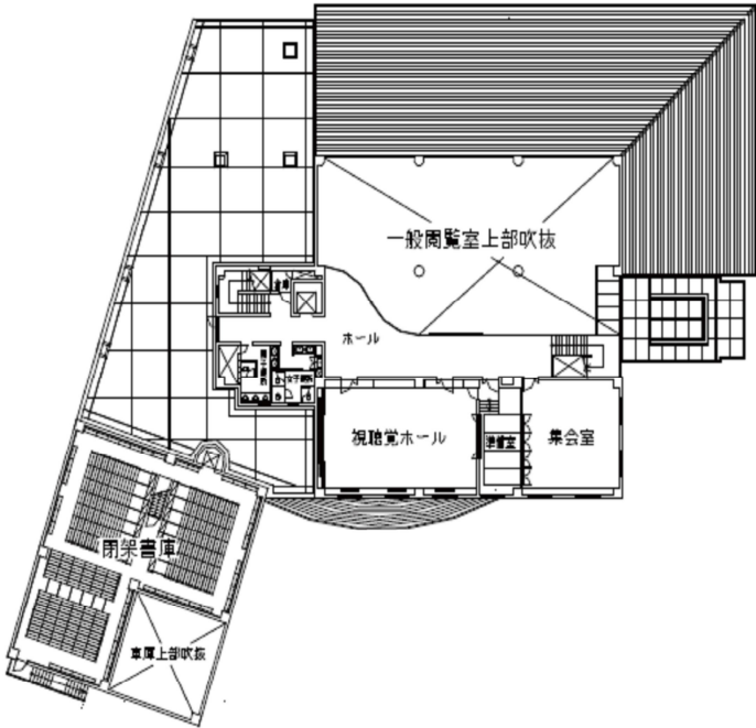
2 階
