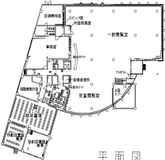
1 階
